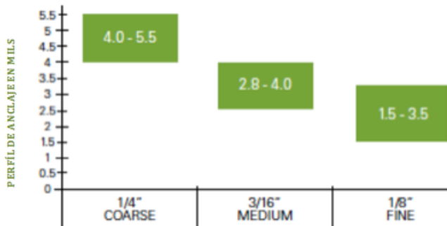
TAMAÑO MÍNIMO DE BOQUILLA VS TAMAÑO DEL GRANO DE CRASHED GLASS
