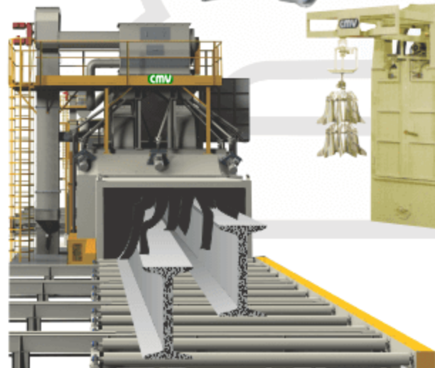
Granalladora con Transportador de Rodillos para Placas y Perfiles Roller Conveyor Shot Blast Machine
